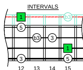
C major-minor arpeggio SEMITONOMETER
